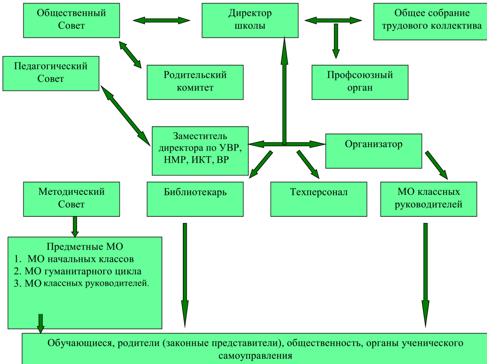
Приложение № 1 Структура управления школой
